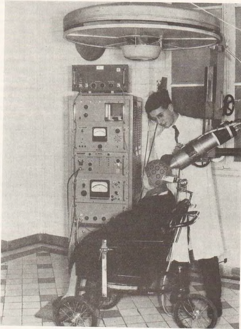
FIG. 6. — Détection préopératoire. Méthode manuelle. Le compteur, perpendiculaire à la surface du crâne, est placé successivement sur chacune des positions figurées d'avance.
